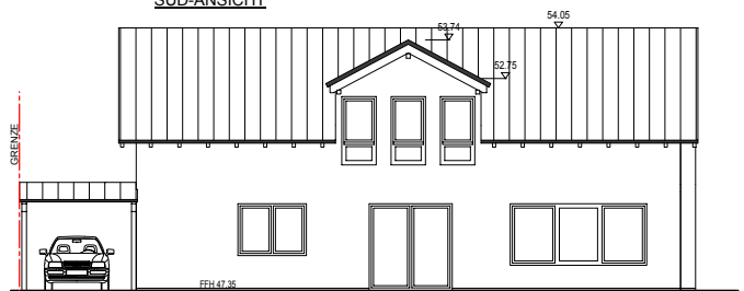
SÜD-ANSICHT
